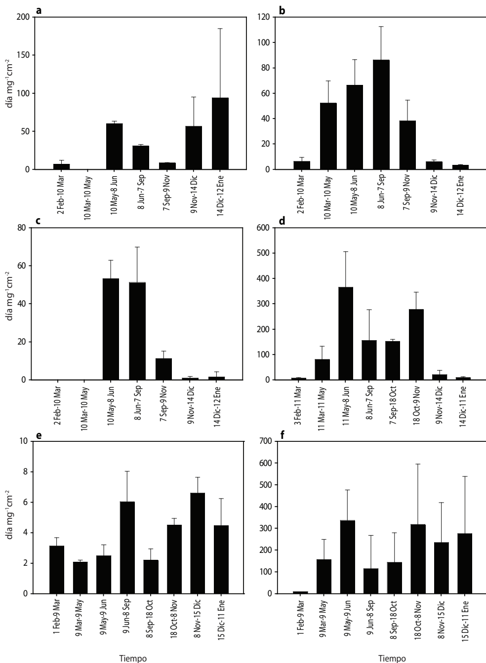
Fig. 1. Tasa de sedimentación (mg cm -2 día -1 ± DE) durante un ciclo anual (febrero 2006-enero 2007) en el área de Bahías de Huatulco. a = San Agustín, b = Jicaral-Chachacual, c = Dos Hermanas, d = Isla Cacaluta, e = La Entrega, f = Isla Montosa. Note las diferentes escalas de los ejes verticales.
